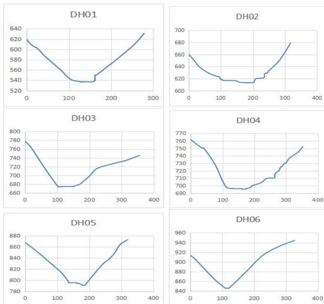
图 4.1-1 监测断面实测大断面示意图见
