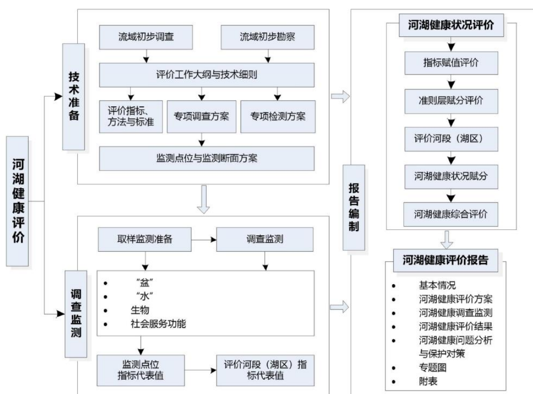
图 1.5-1 朝天区清边河河流健康评价工作流程图
